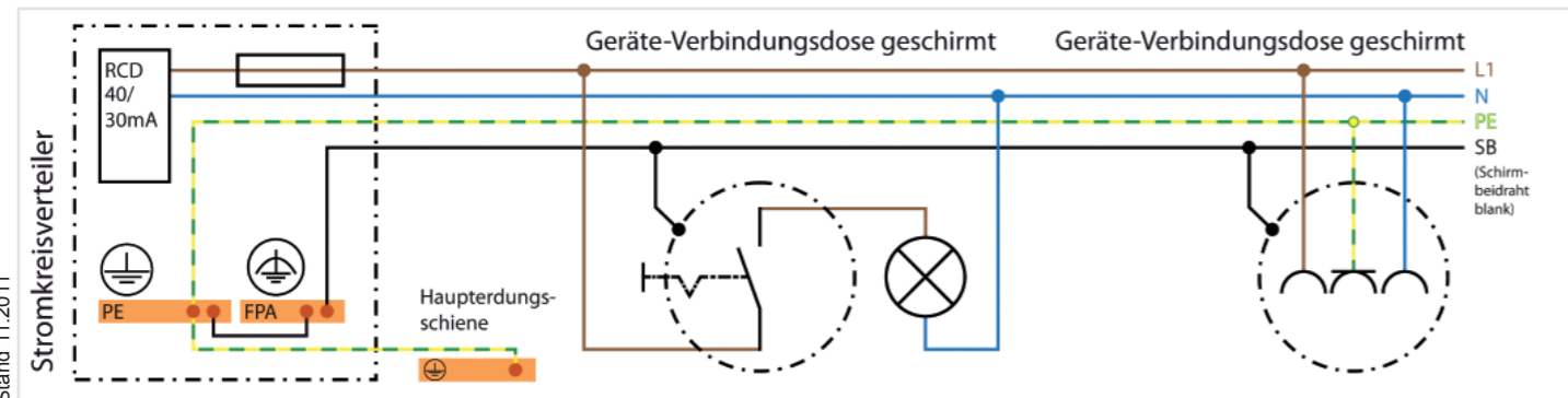
Bild 1: Verdrahtungsschema „Geschirmte Elektroinstallation“
