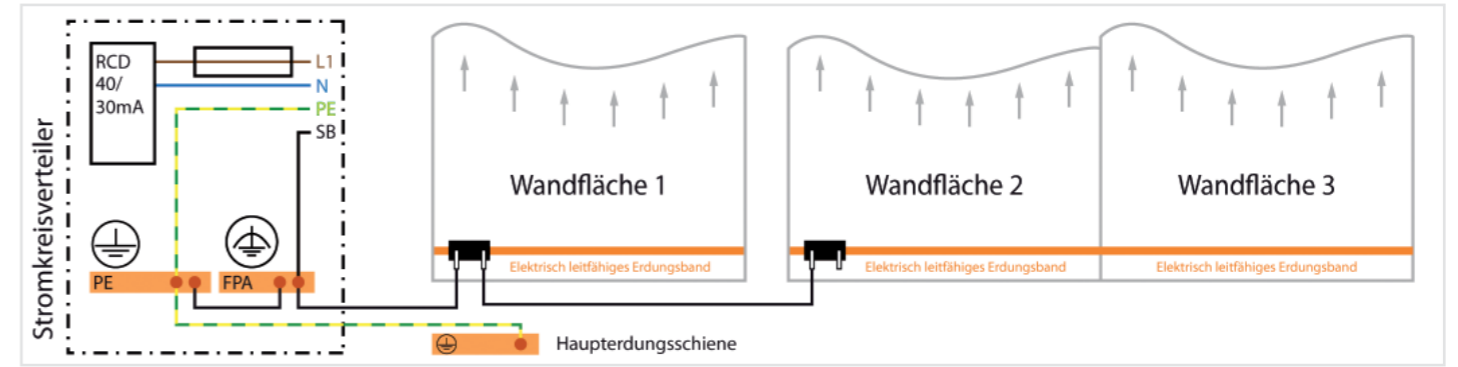
Bild 5: Verdrahtungsschema „Großflächige Abschirmungen“
